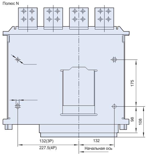
Размеры отверстий в основании
